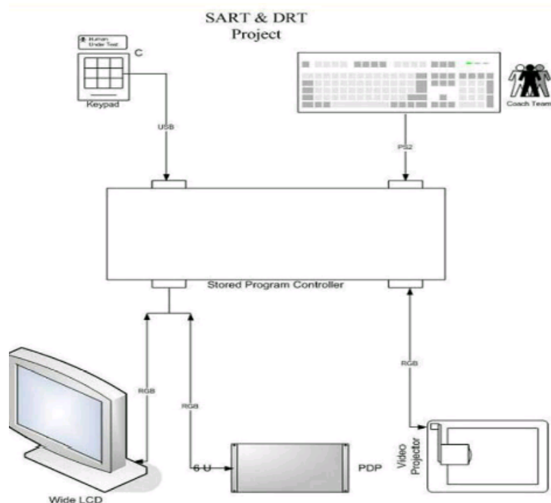
تصویر ۱: اجزای مختلف سامانه
