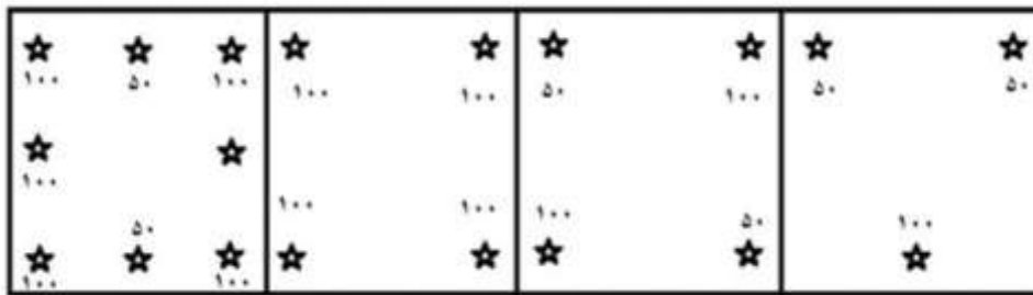
تصویر ۱. نحوه آرایش فنرها زیر سطح. عدد نشان‌دهنده میزان سفتی فنر مورد نظر است
